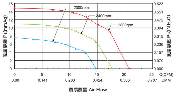
風量, 靜壓特性曲線 風量, 靜圧特性カーブ Characteristic Curves
