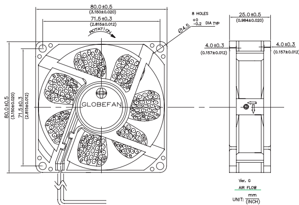
外形圖 外形図 Outline
