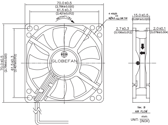
外形圖 外形図 Outline
