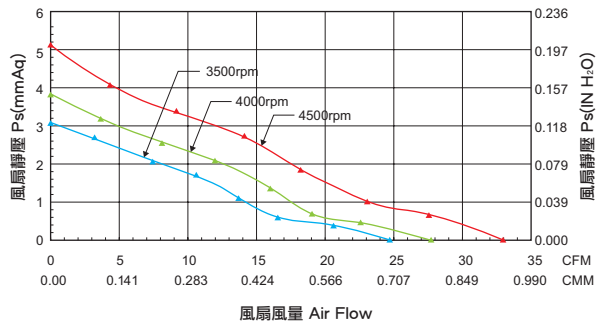
風量, 靜壓特性曲線 風量, 靜压特性カーブ Characteristic Curves
